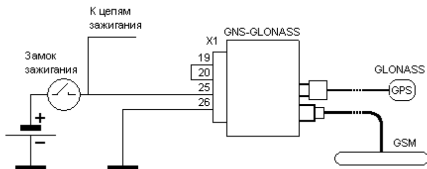
Рис. 8. Простейший вариант подключения прибора к цепям зажигания автомобиля
