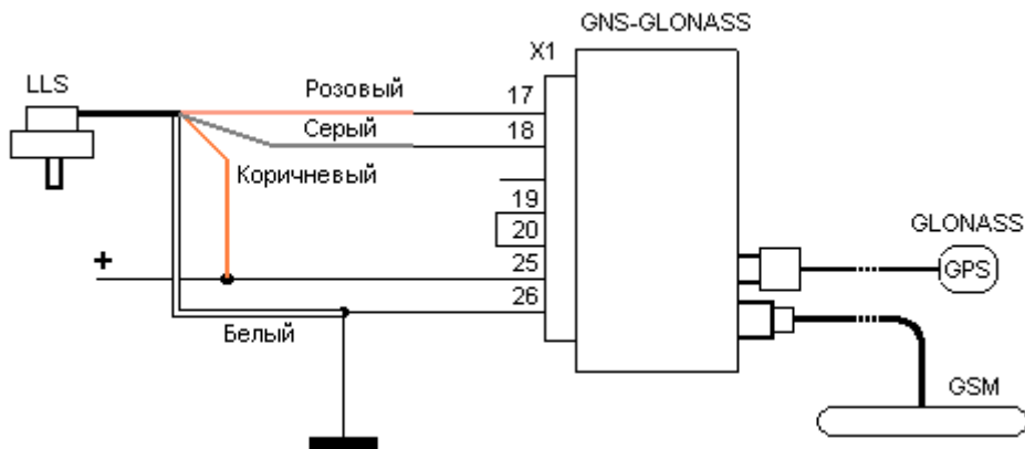
Рис. 14. Пример подключения датчика уровня топлива LLS к прибору
