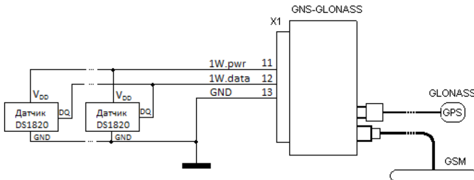
Рис. 15 Пример подключения температурных датчиков к прибору
