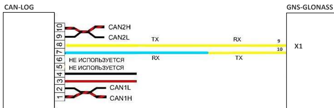
Рис.16 Схема подключения прибора через CAN-LOG к CAN-шине автомобиля
