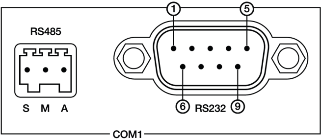
Рис. 10. Внешний комбинированный порт
