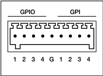
Рис. 8. Интерфейсный разъём
