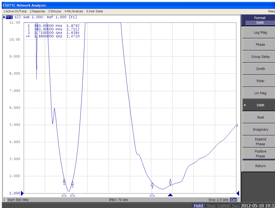
< VSWR >
