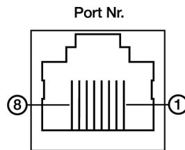
Рис. 6. Ethernet-разъем
