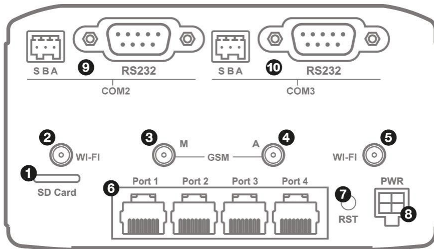
Рис. 2. Вид сзади RL25w
