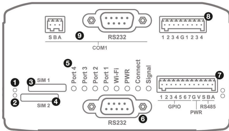
Рис. 3. Вид спереди RL25w
