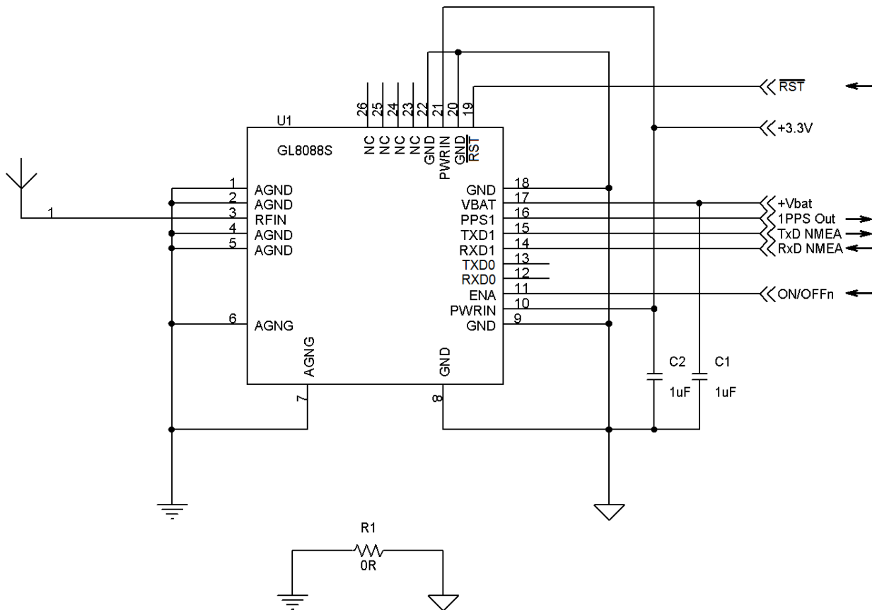
Рис.5. Типовая схема включения приемника GL8088s.
