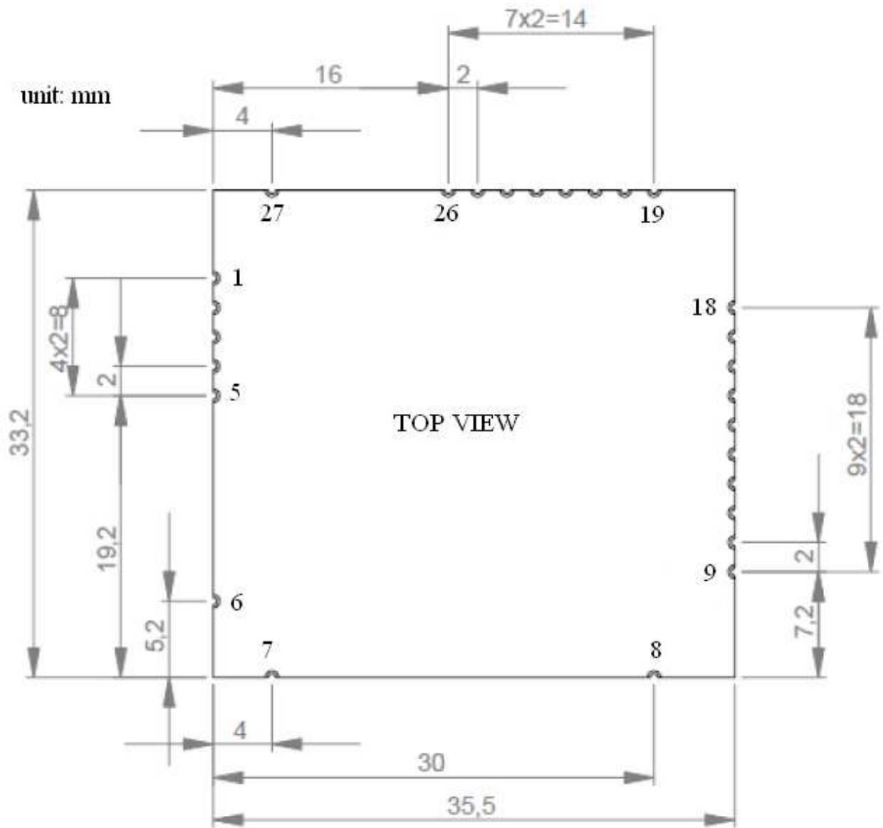
Рис.3. Габаритно-присоединительные размеры приемника GL8088s.
