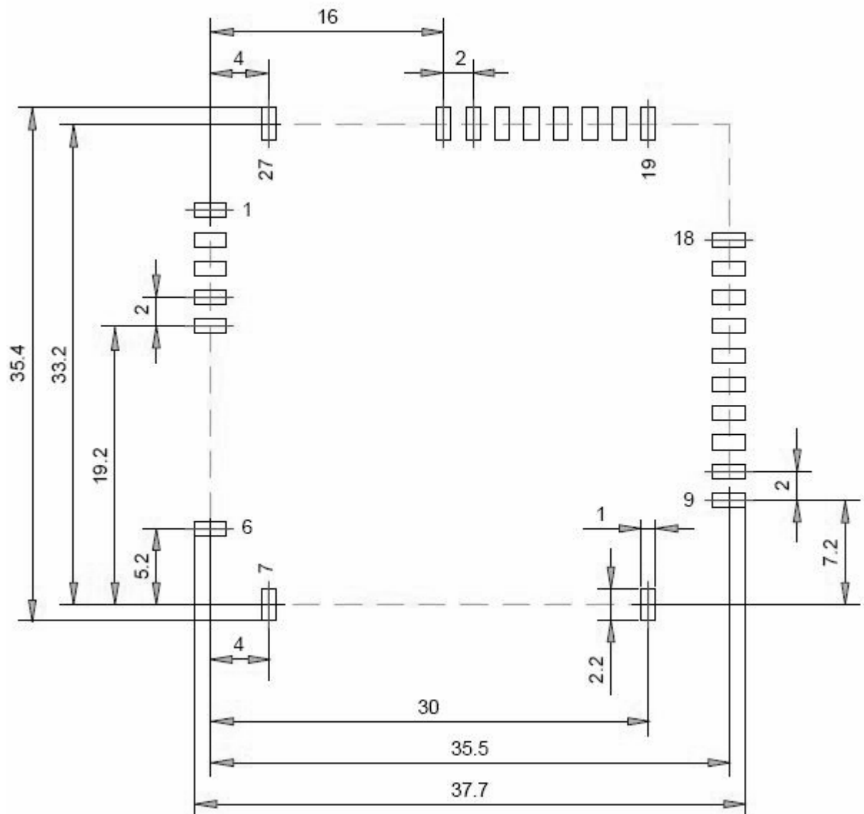
Рис.4. Рекомендуемое посадочное место для установки приемника GL8088s.
